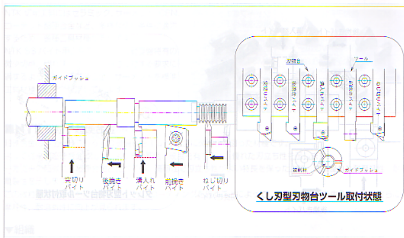
小型 CNC 自動旋盤(くし刃型)ツーリング例
